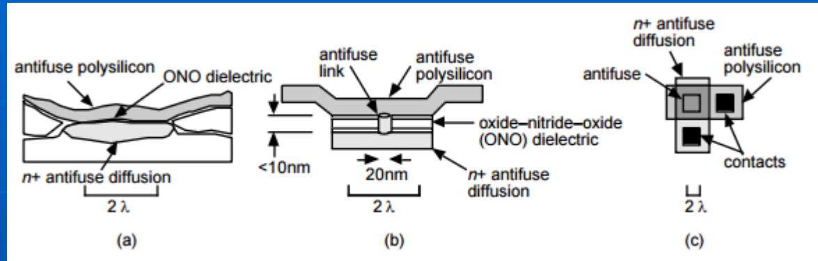
Vista realística del antifusible. Vista esquemática en profundidad. Vista esquemática superior.
